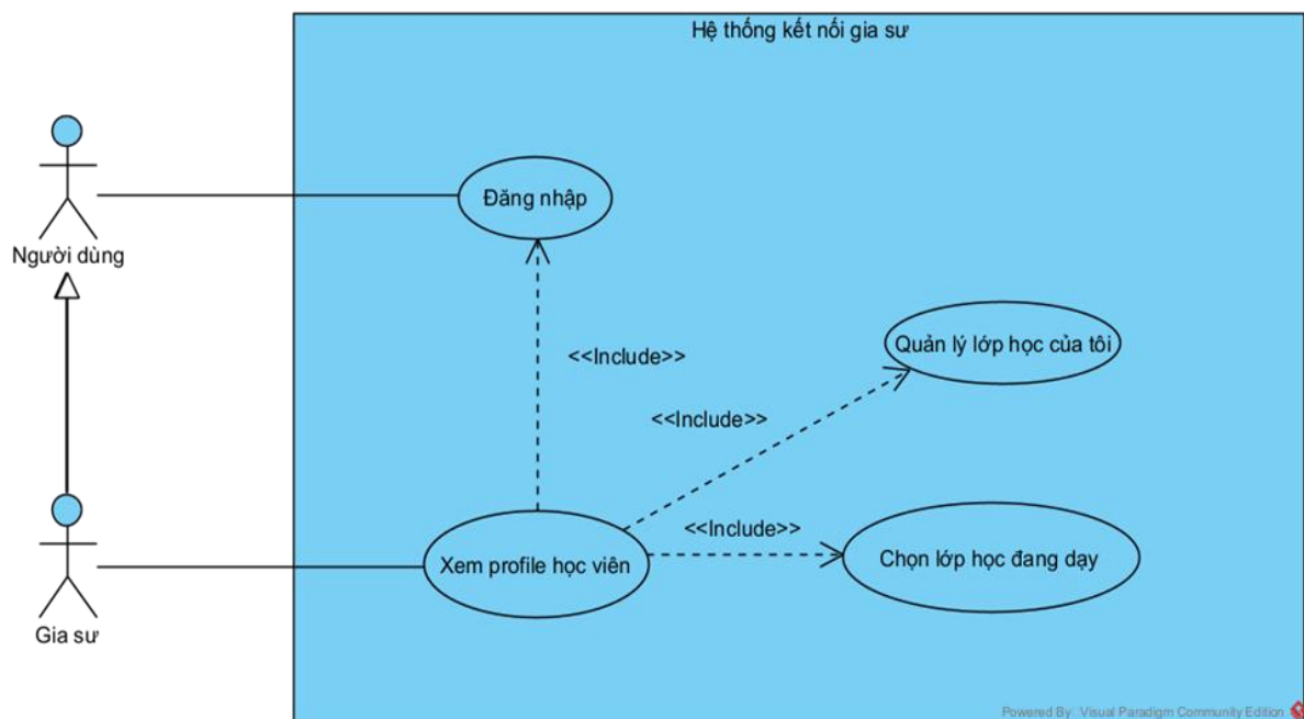
Hình 2.4. Biểu đồ use case chức năng xem profile học viên
