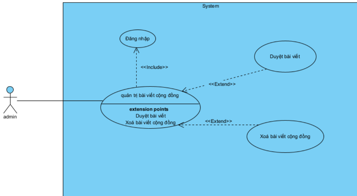
Hình 2.24. Biểu đồ use case chức năng quản lý bài viết cộng đồng
