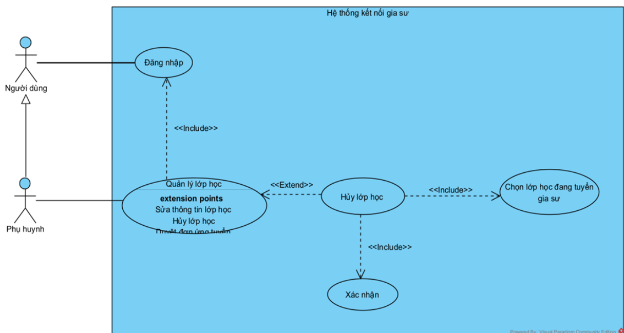
Hình 2.12. Biểu đồ use case chức năng hủy lớp học
