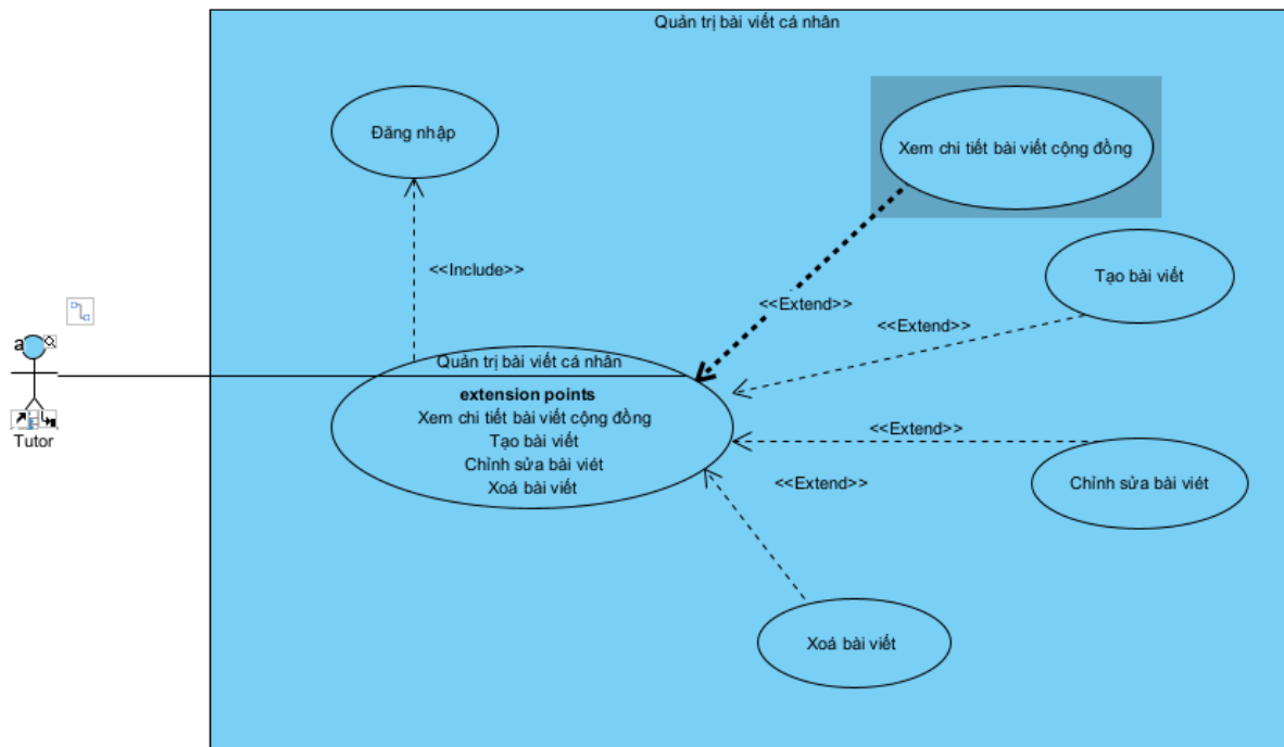
Hình 2.23. Biểu đồ use case chức năng quản lý bài viết cá nhân
