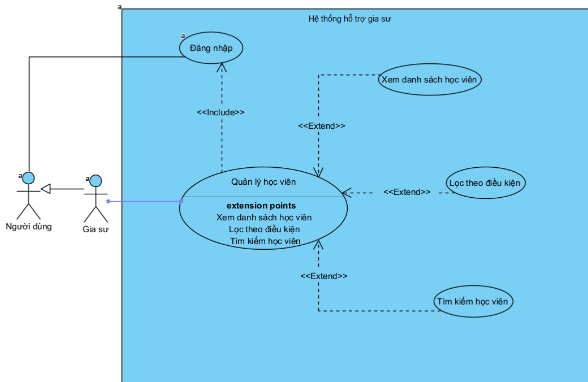
Hình 2.20. Biểu đồ use case chức năng quản lý học viên
