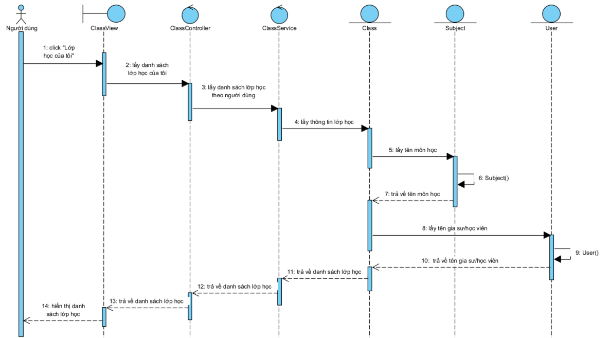
Hình 2.44 Biểu đồ tuần tự chức năng Xem danh sách lớp học
