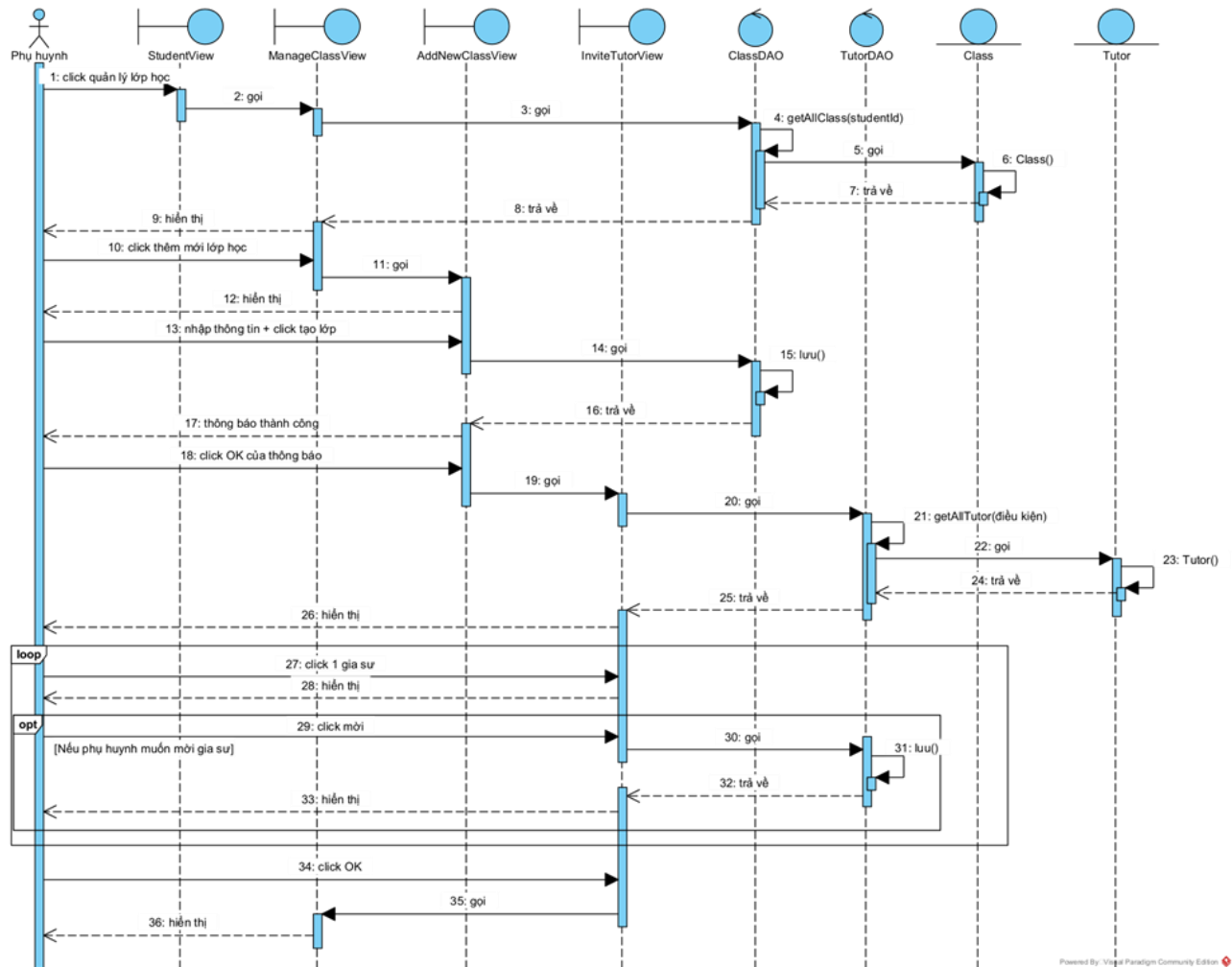
Hình 2.37 Biểu đồ tuần tự chức năng Tạo lớp học
