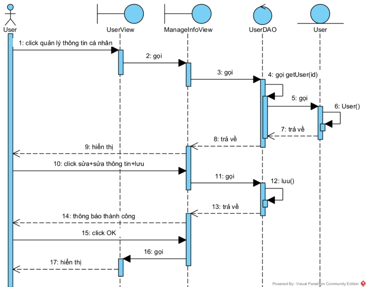
Hình 2.30 Biểu đồ tuần tự chức năng Quản lý profile gia sư
