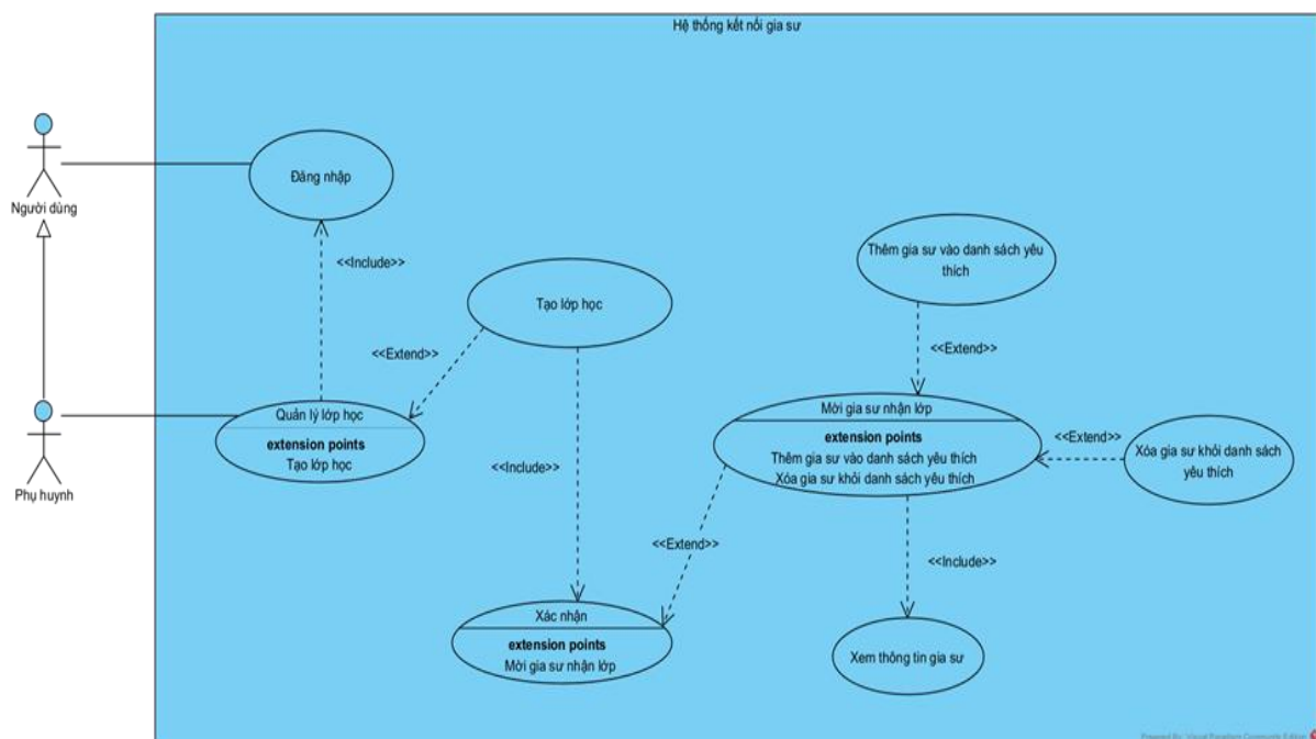
Hình 2.10. Biểu đồ use case chức năng tạo lớp học
