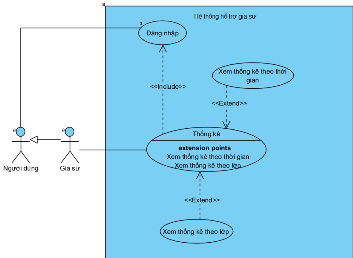
Hình 2.21. Biểu đồ use case chức năng thống kê
