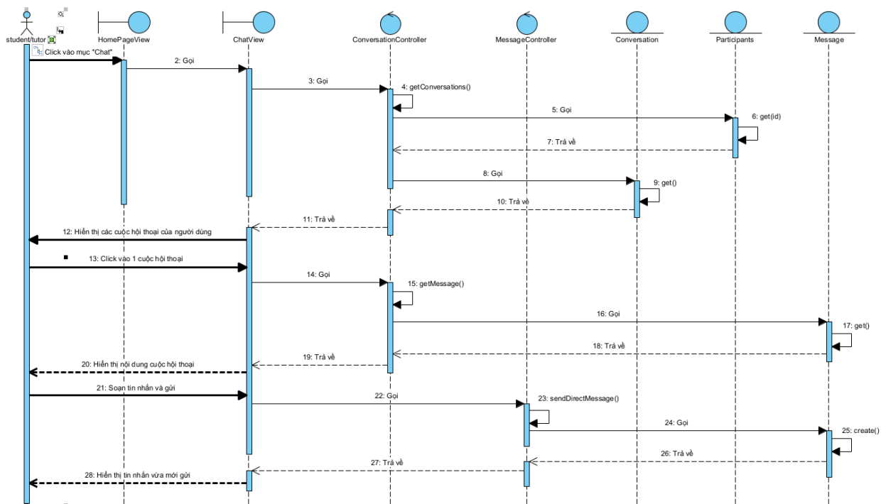
Hình 2.67 Biểu đồ tuần tự chức năng Chat
